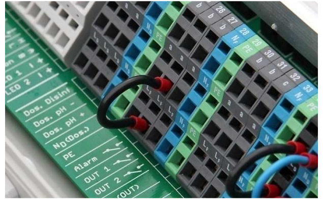
Drahtbrücke im Klemmraum von der Phase L F auf den Mittelkontakt a
